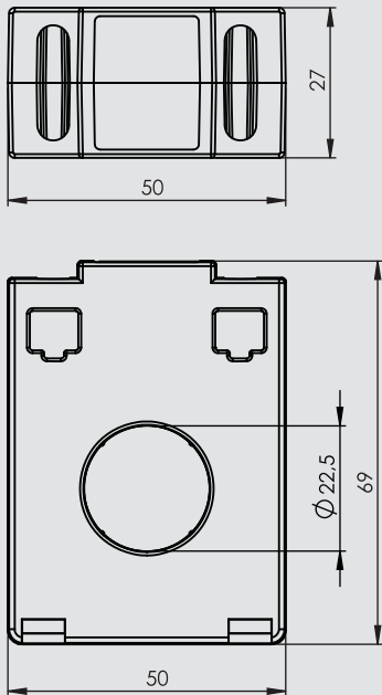
Teknik Resim
